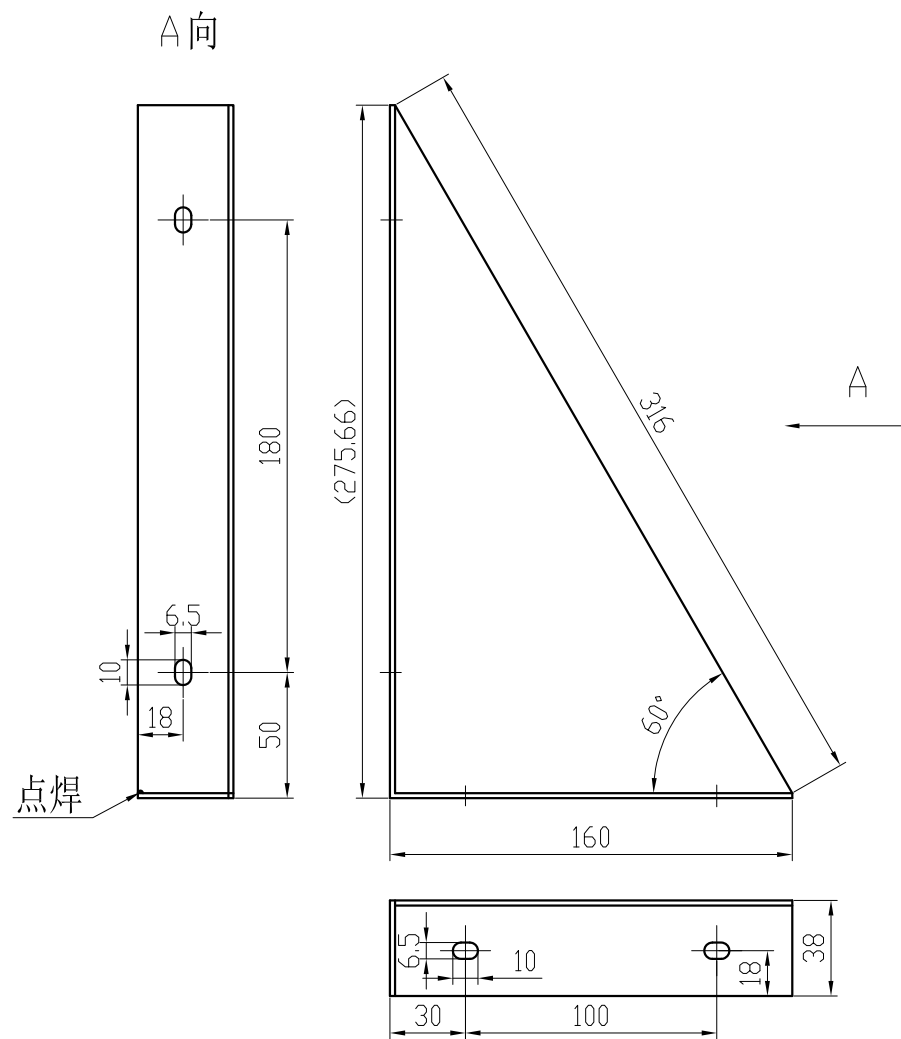
折弯图
